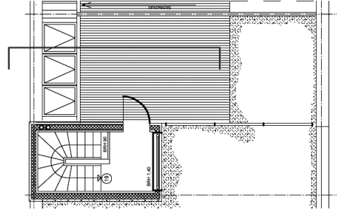
2.OG / Dachterrasse
