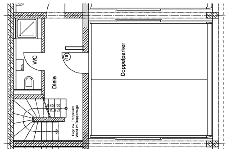
KG / Tiefgarage
