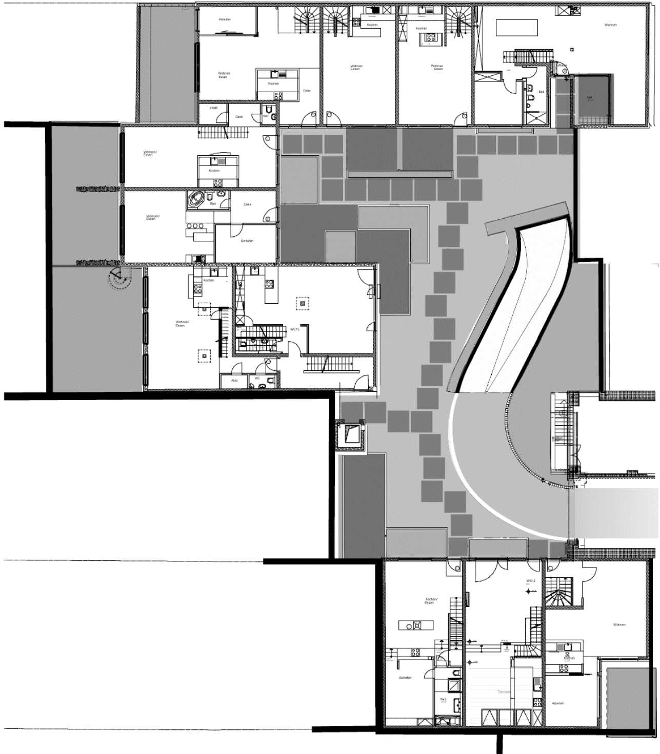
Grundriss EG, mit Außenanlage
