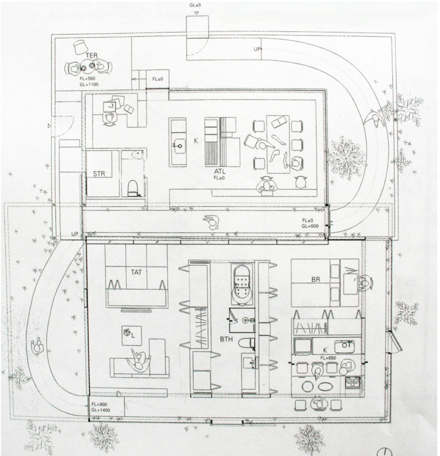
Plan S=1:150
