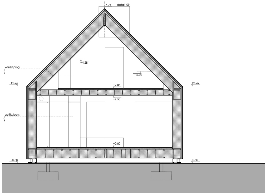
snede C_C: nieuwe toestand
