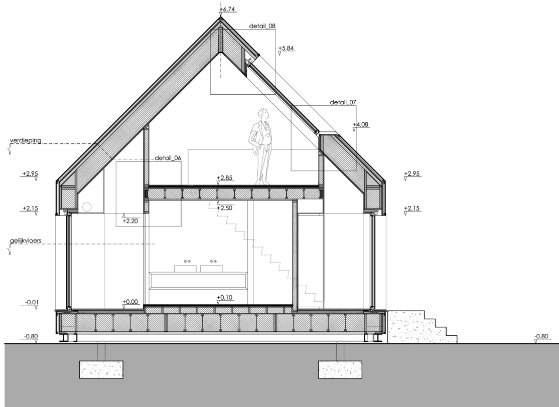
snede B_B: nieuwe toestand
