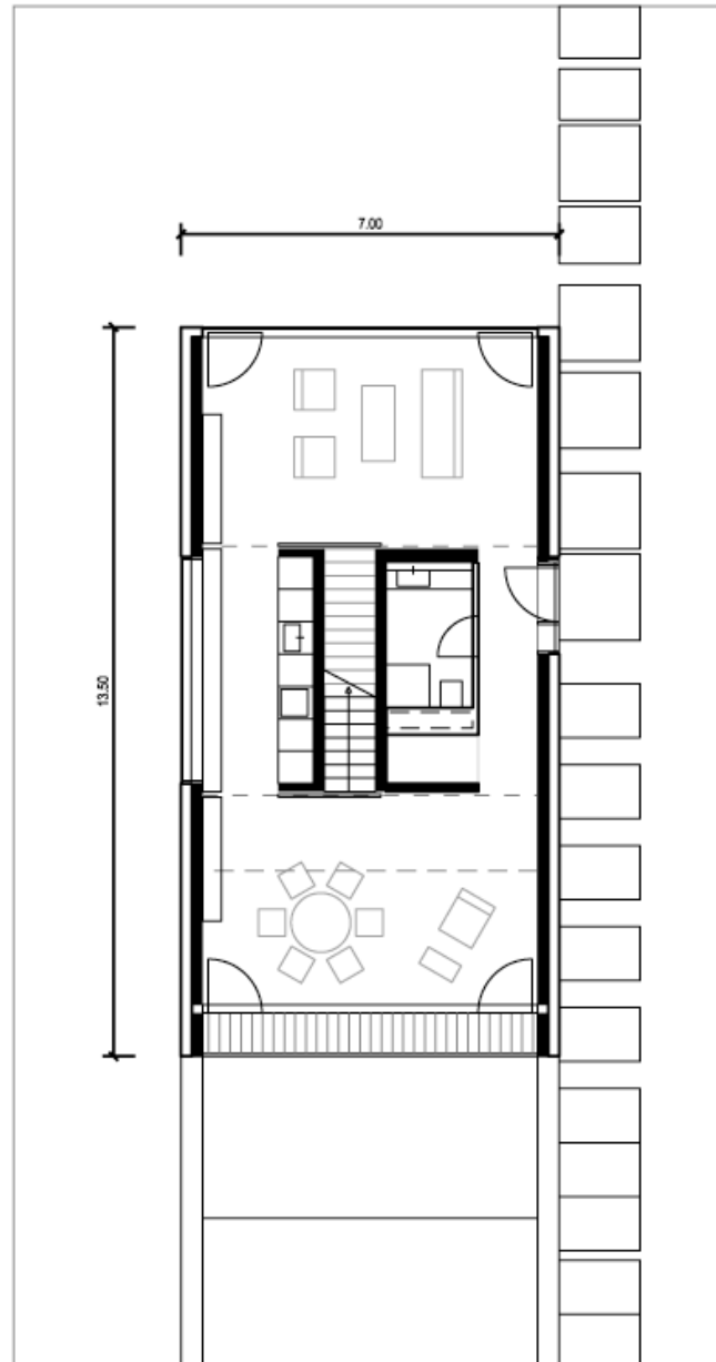
ERDGESCHOSS
