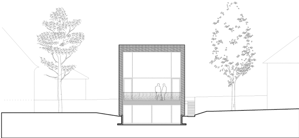
ANSICHT OST
