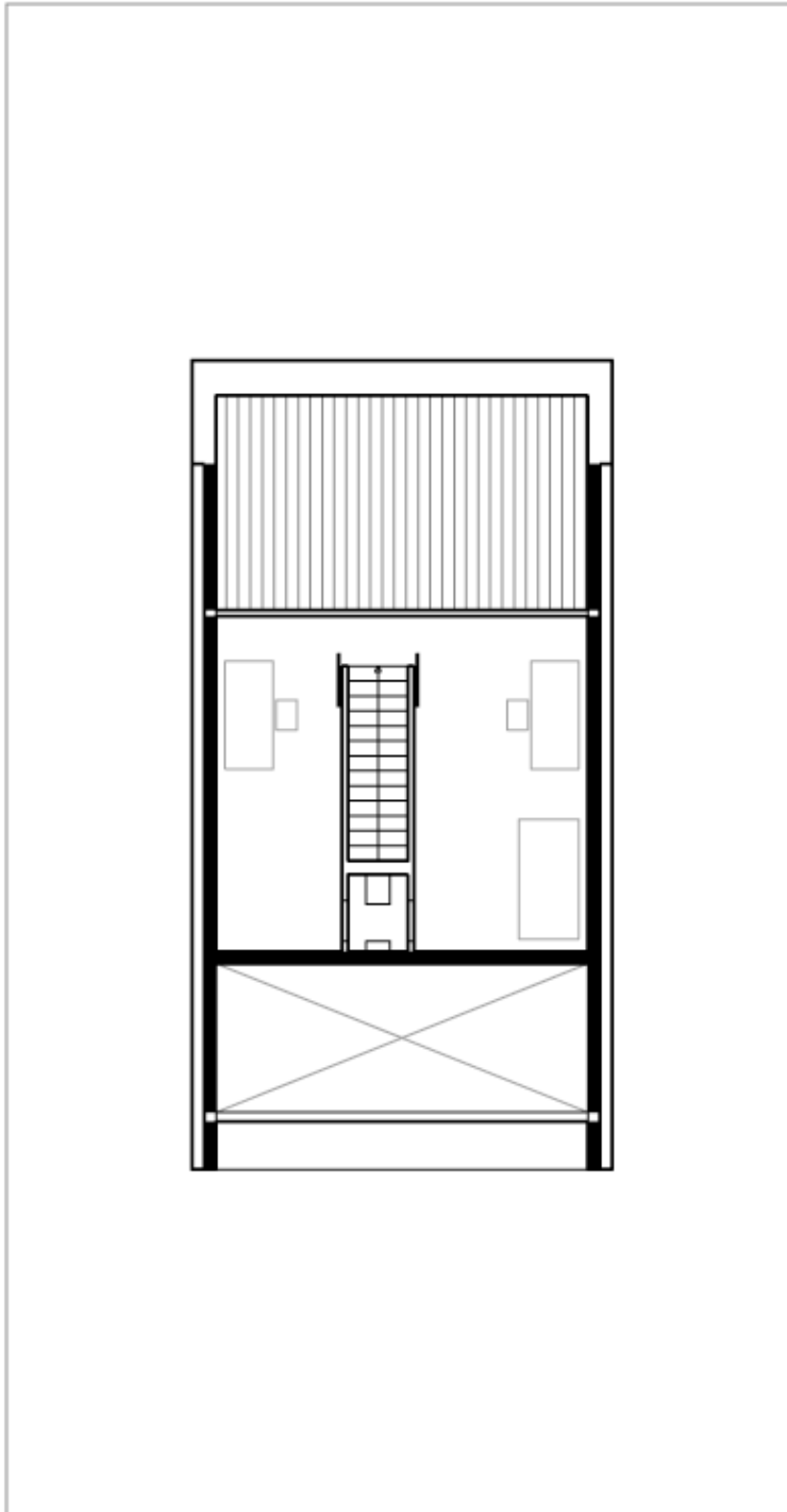
OBERGESCHOSS
