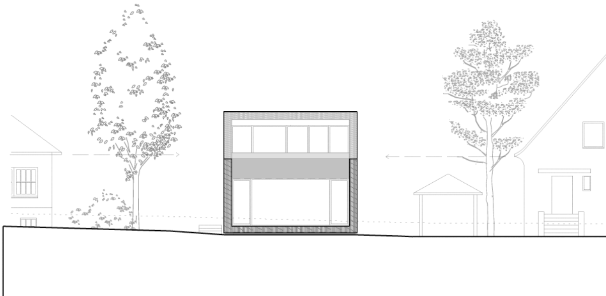
ANSICHT WEST
