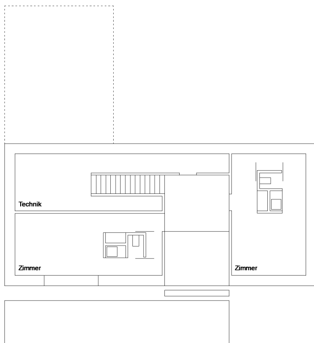
Niveau -2
