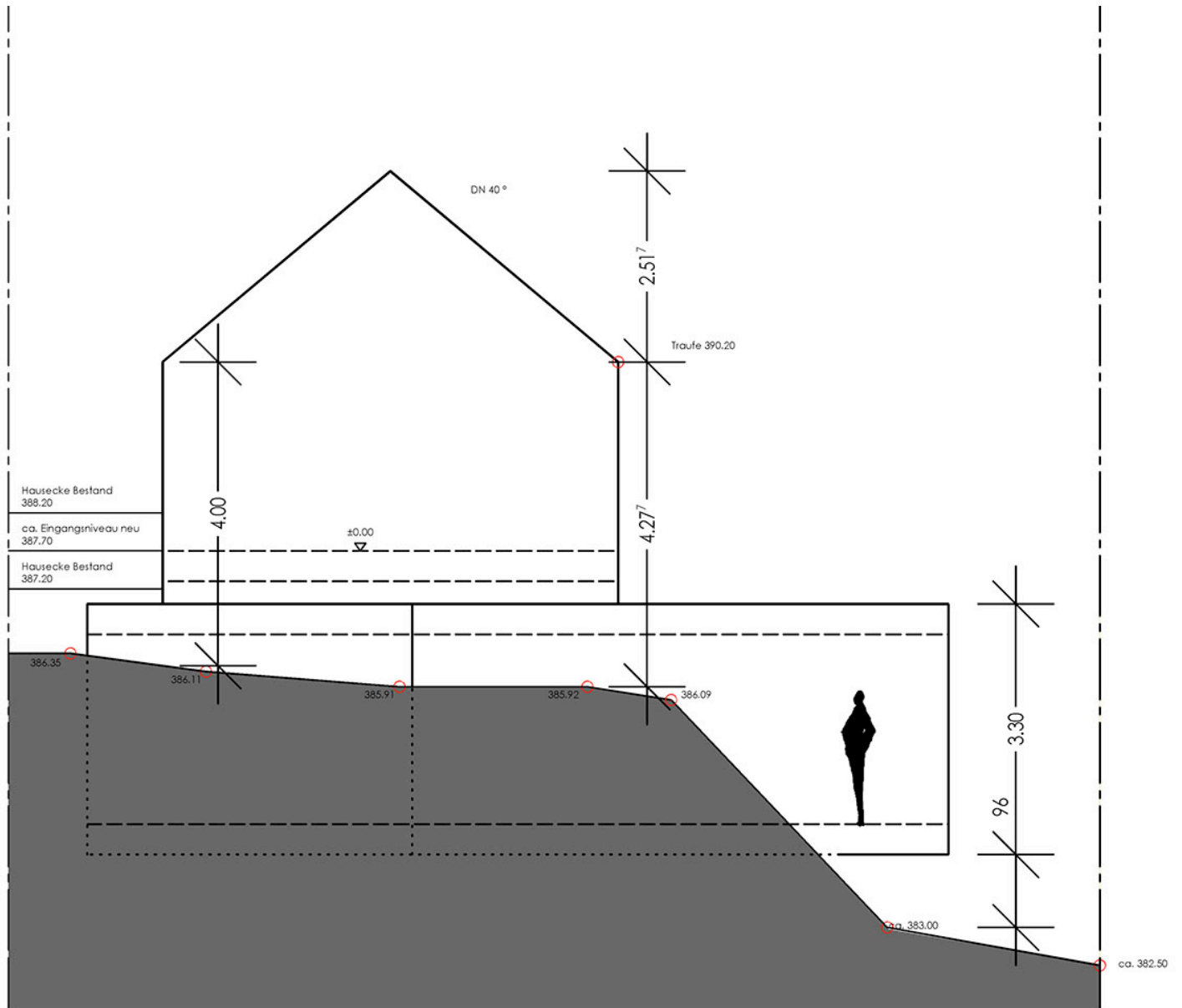
Schnitt 1
