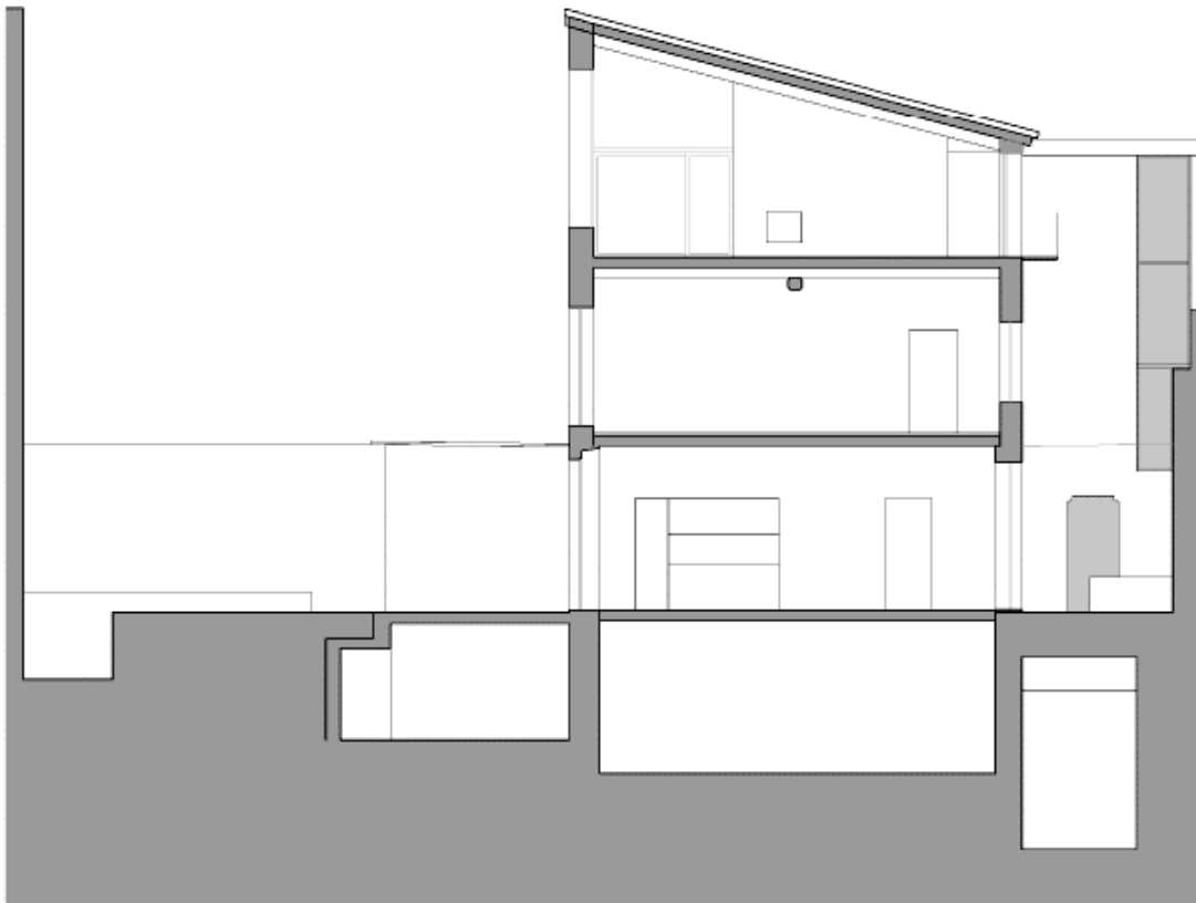
LONGITUDINAL SECTION
