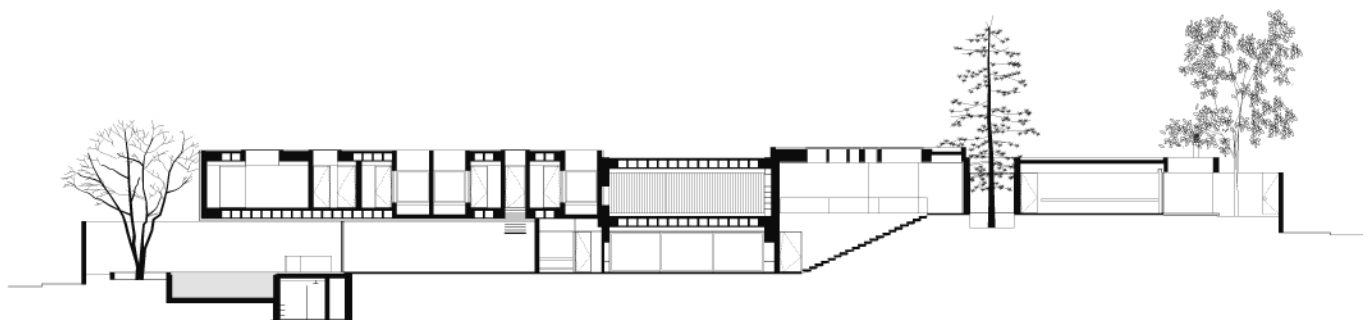
LONGITUDINAL SECTION 0 5 m
