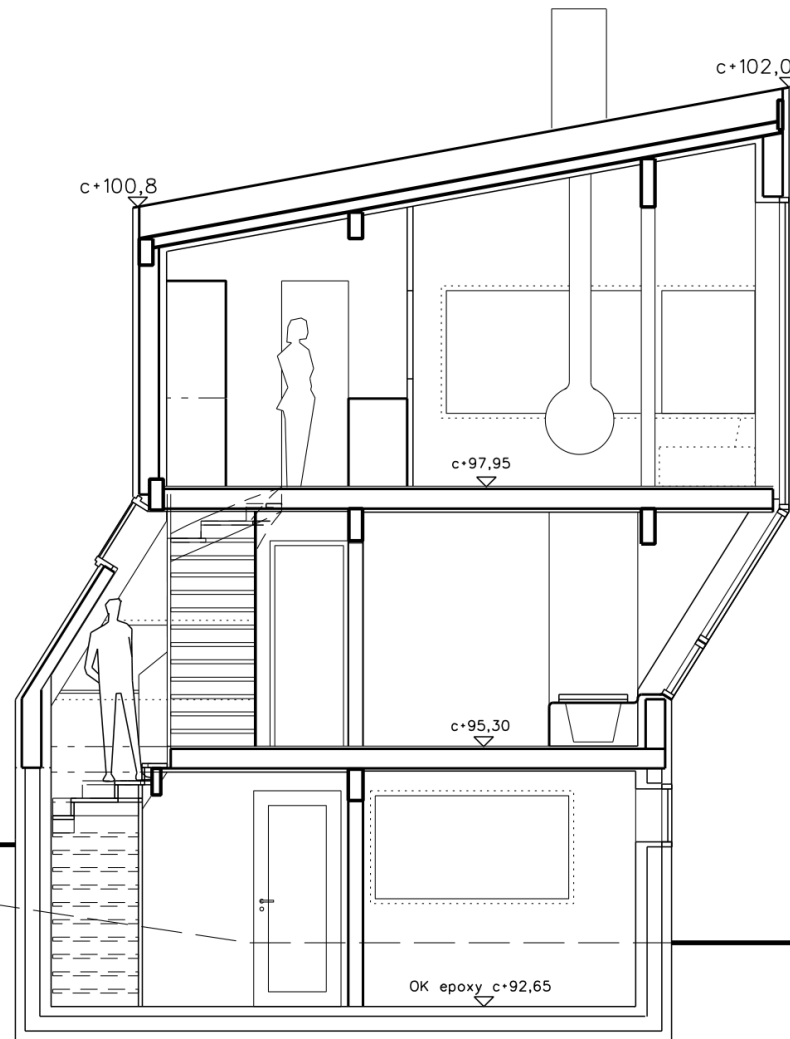
SECTION A-A
